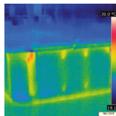
Verifica di perdita di calore con sistema Nordic Insulation System
